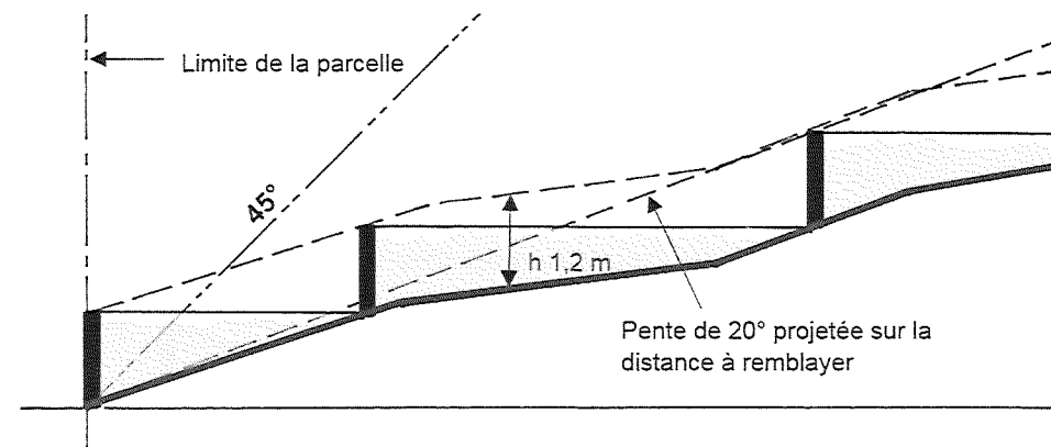
Remblayages avec mur de soutènement
